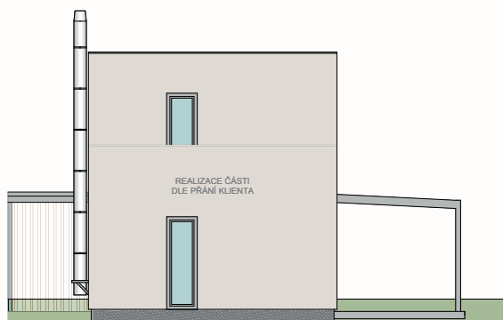
FASÁDA SEVEROVÝCHODNÍ
