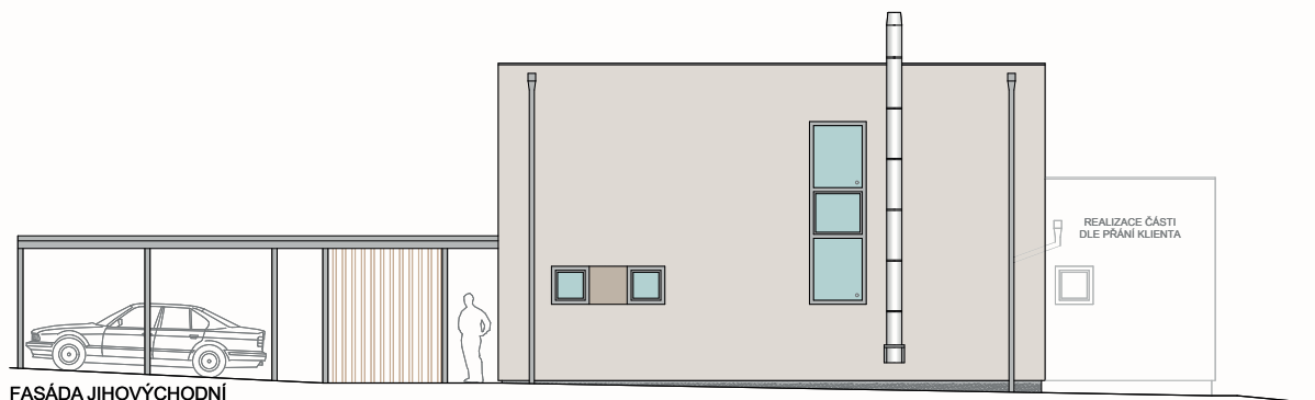
FASÁDA JIHOVÝCHODNÍ
